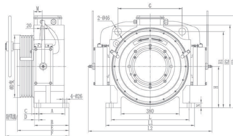
外观尺寸图 | Outline drawing
