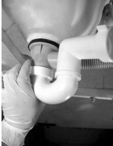
نصب سیفون
